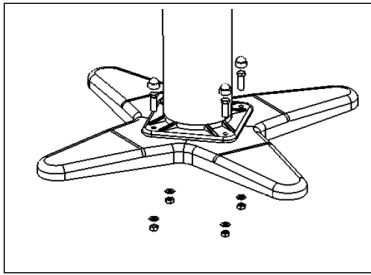
1. ábra Az állvány összeszerelése
